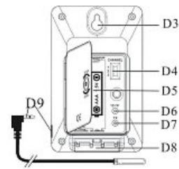
RÜCKANSICHT
